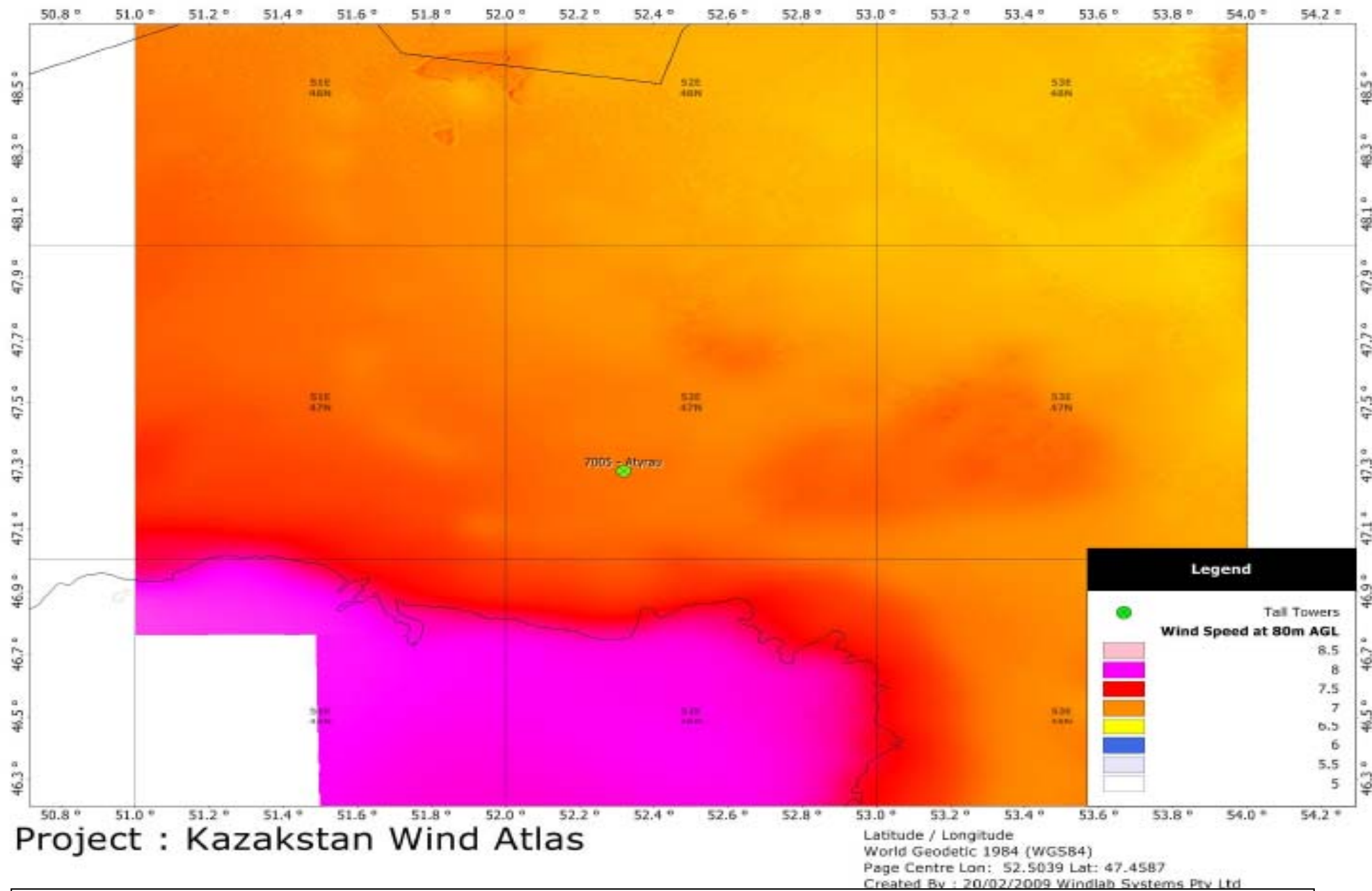
Рис. 2. Ветровая карта участка в районе Атырау на высоте 80 м над уровнем земли и разрешением 100 м.
